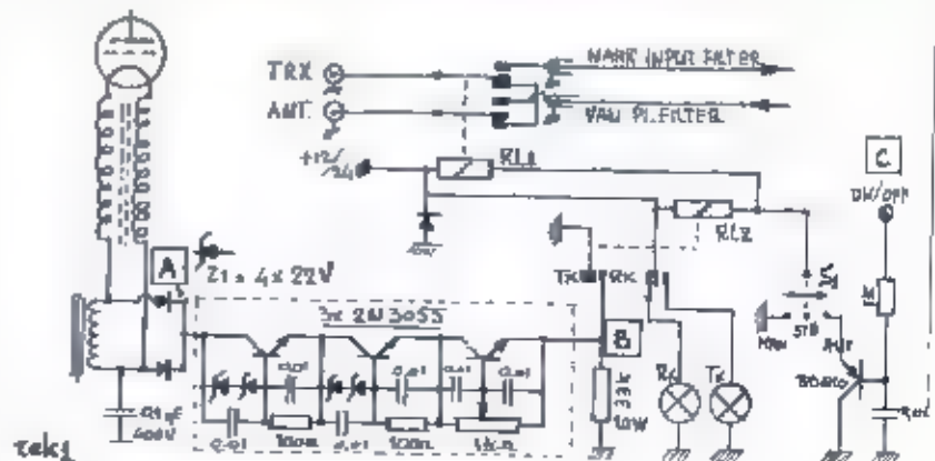
Tekening 1: Schema van de voorinstelling en de relais
